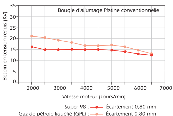
fig.1 Besoin en tension d'une bougie en fonction du carburant
