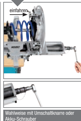
Betätigen
