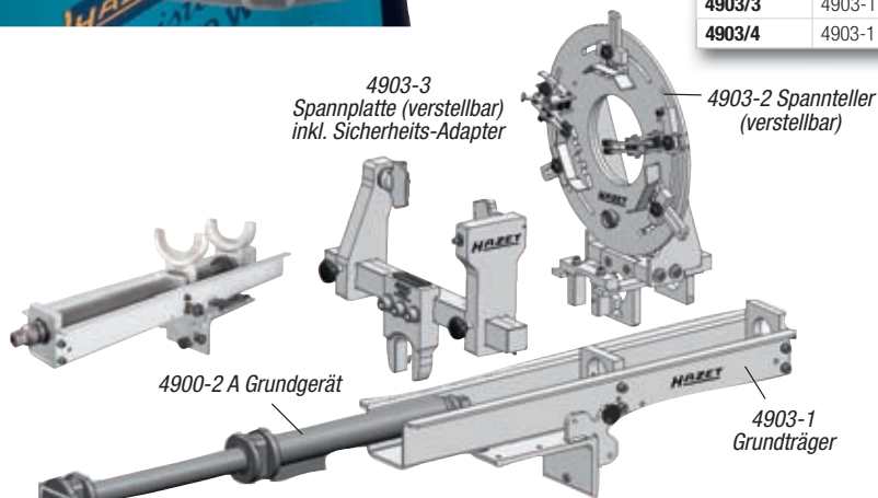
Federbein-Fixierung
